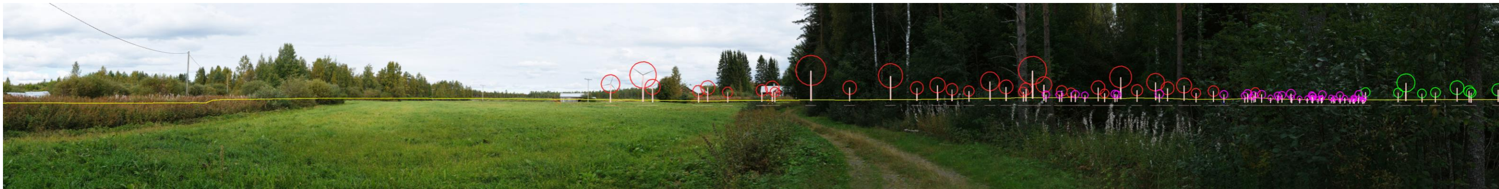
Kuva 19. Kuvauspiste 5 (Maaralanperä), havainnekuvaluonnos vaihtoehdossa VE 1. Etäisyys lähimpään Konnunsuon voimalaan on noin 2,9 kilometriä
