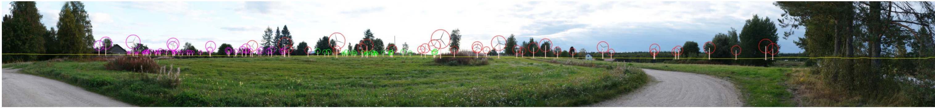
Kuva 3. Kuvauspiste 1 (Ahokylä), havainnekuvaluonnos vaihtoehdossa VE 1. Etäisyys lähimpään Konnunsuon voimalaan noin 2,5 km.
