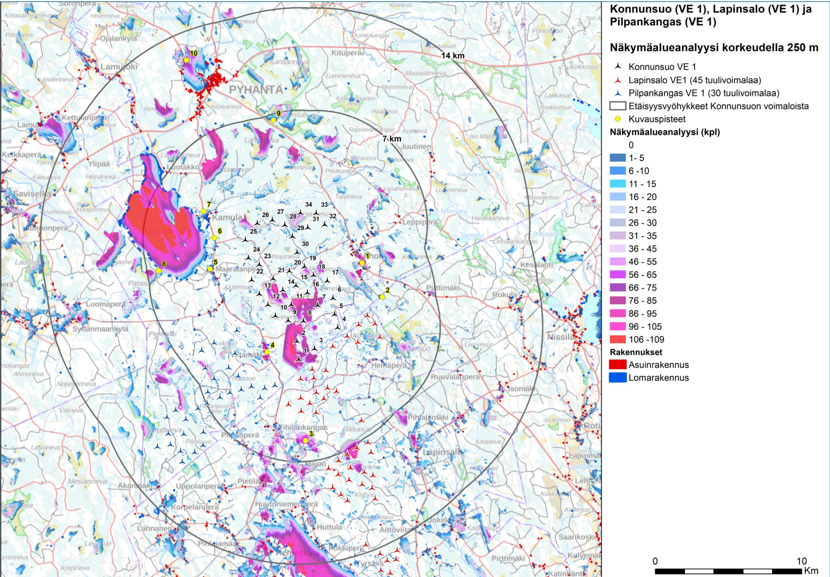
Kuva 1. Konnunsuon tuulivoimahankkeen tuulivoimapuiston näkymäalueanalyysin laskentatulokset hankevaihtoehdossa VE 1 lavan puoliväliin (HH +1/4 RD) mallinnettuna.
