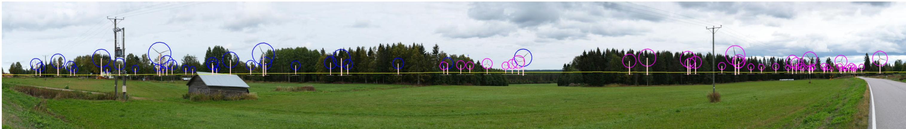
Kuva 17. Kuvauspiste 4 (Viitamäki), havainnekuvaluonnos vaihtoehdossa VE 2. Etäisyys lähimpään Konnunsuon voimalaan on noin 3,2 kilometriä.
